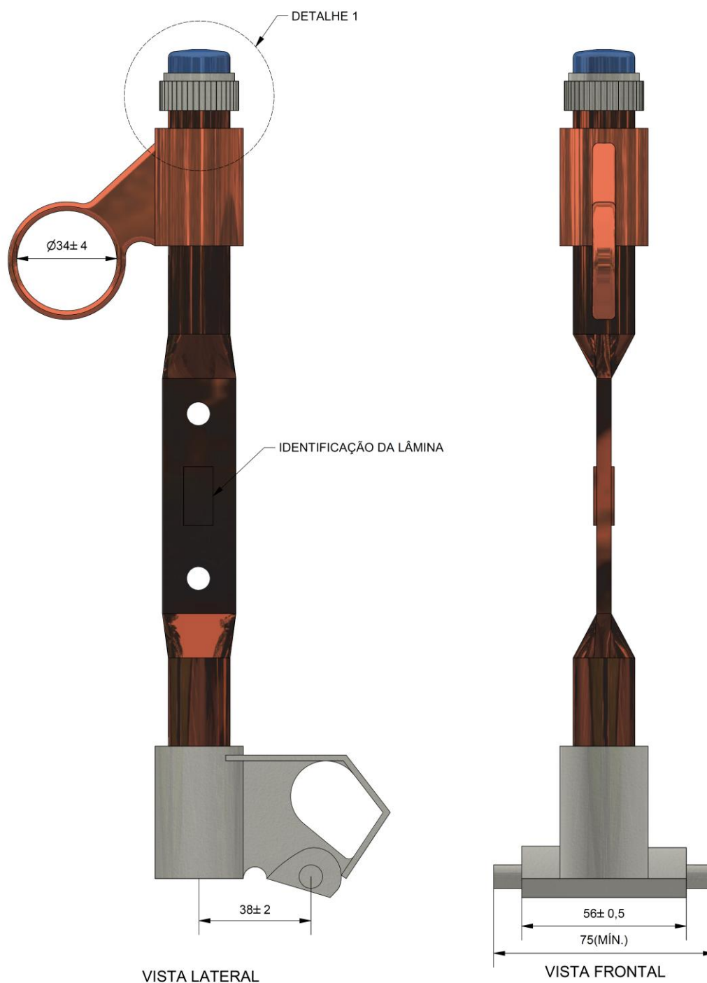
Figura 1 - Lâmina desligadora
